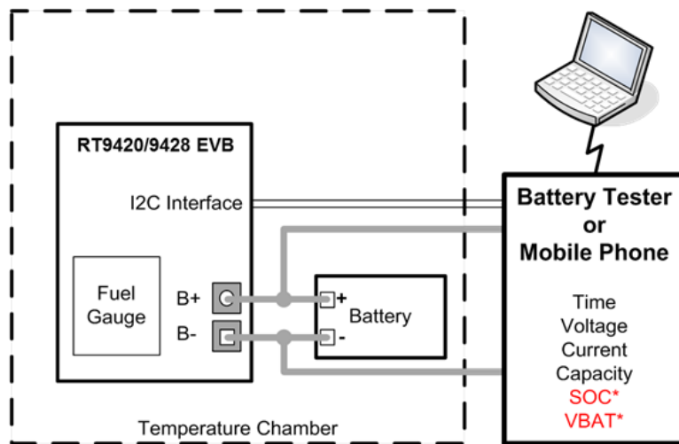
圖十八、從電量計透過 I 2 C 界面和測試器或手機存取 SOC，VBAT
