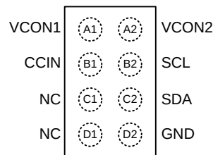
WL-CSP-8B 0.96x1.64 (BSC)
