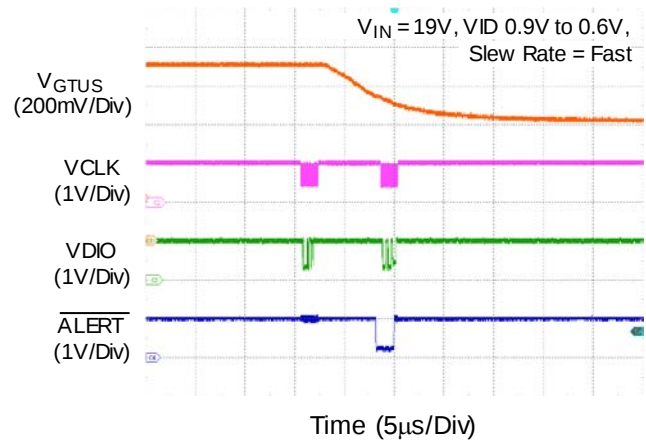
GTUS VR Dynamic VID Down
