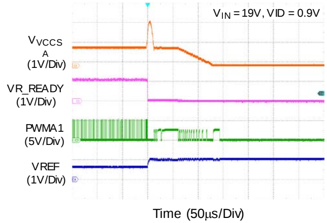
VCCSA VR OVP
