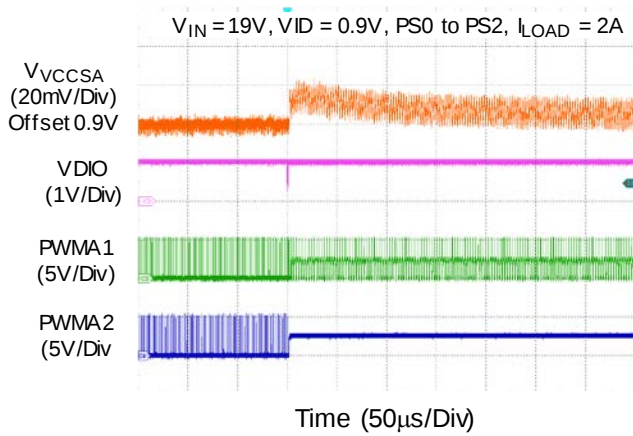
VCCSA VR Mode Transient
