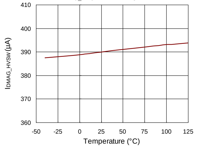
I_{DMAG\_HVS} vs. Temperature
