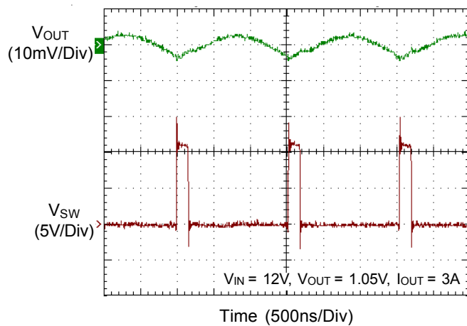
VOUT Ripple
