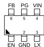
T/SOT-23-6
