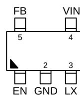
T/SOT-23-5
