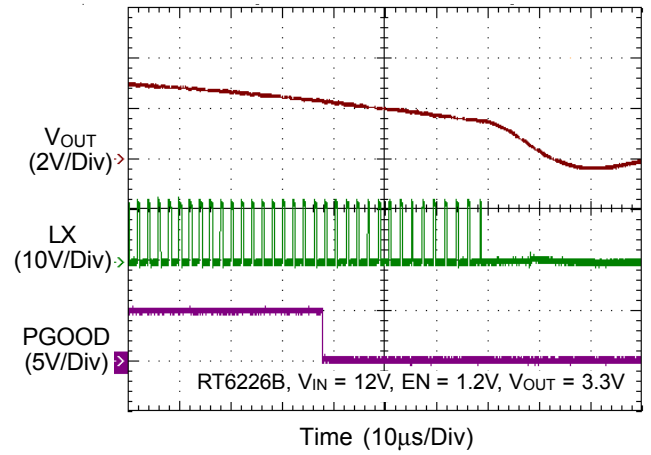
VOUT UVP
