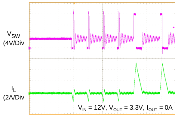
BOOT UVLO
