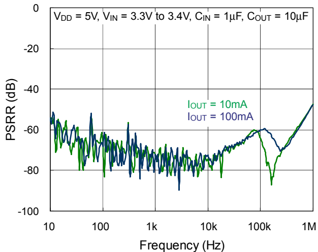
PSRR
