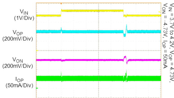
V OP Line Transient
