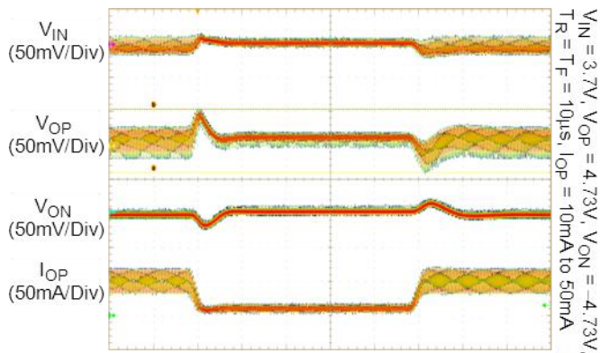
V OP Load Transient
