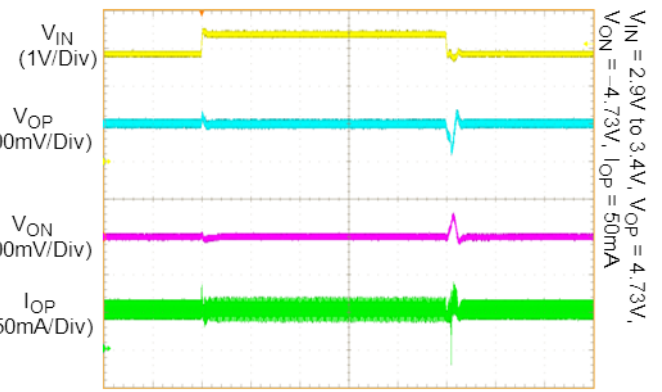
V OP Line Transient
