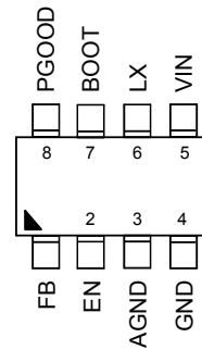
TSOT-23-8 (FC)
