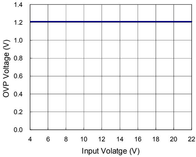
OVP Voltage vs. Input Volatge
