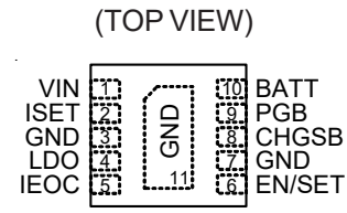
WDFN-10L 3x2
