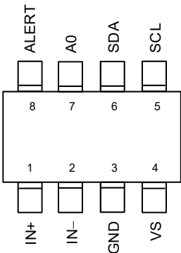
TSOT-28(COL)
