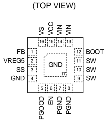
WQFN-16L 3x3
